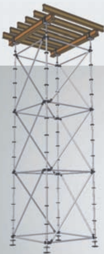
Schema tipo per torre con carico ammissibile di 30 kN per stelo
