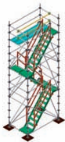
Scala a torre bidirezionale
